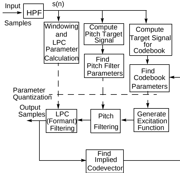
Fig. 1 BI-CELP Encoder
